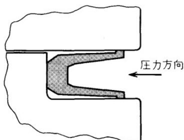
図19 メタルレジリエントシール その特徴は
