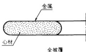
図21メタルジャケット形ガスケット
