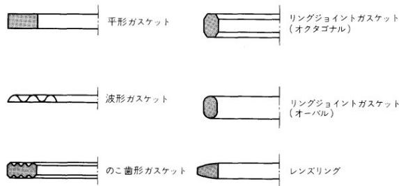
図20 金属ガスケット
